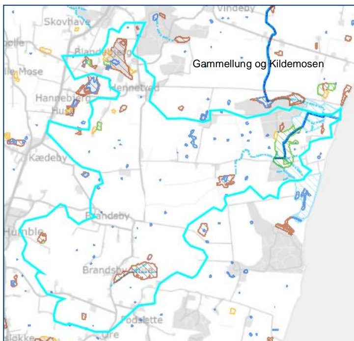
Figur 1. Afløbet fra Frederiksberg og Skovsgårds Enge som ønskes nedklassificeret med åben (blå) strækning inden for oplandet (turkis). Beskyttet natur er vist med skravering.
